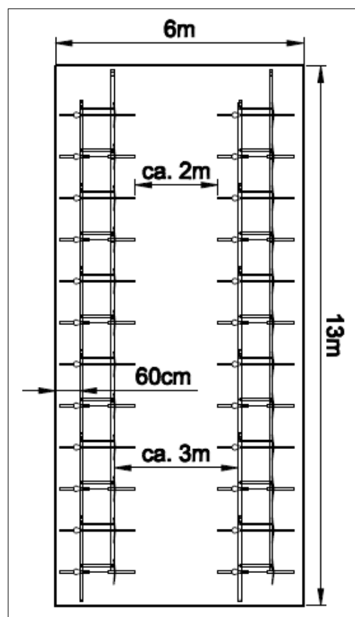
Abb.: radpark für 48 Fahrräder
